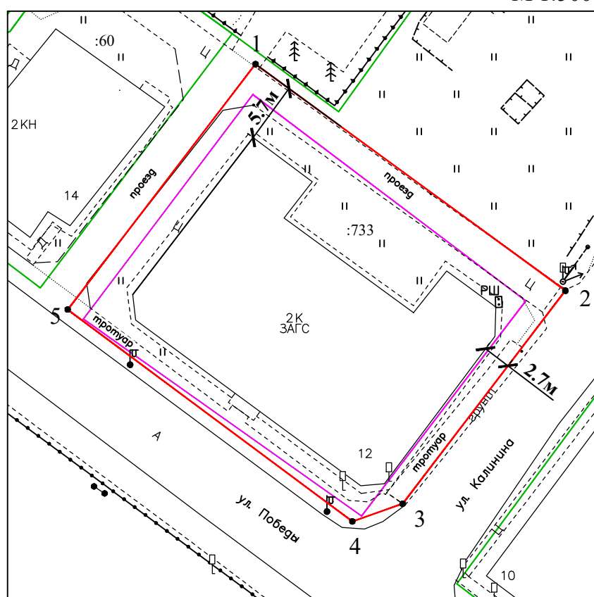
ВЕДОМОСТЬ КООРДИНАТ ПОВОРОТНЫХ ТОЧЕК ПРИЛЕГАЮЩЕЙ ТЕРРИТОРИИ
